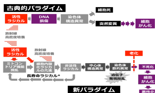
図3 放射線発がんのDNA 損傷起源仮説と非DNA 損傷起源説
