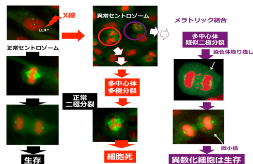
図2 染色体異数化誘導経路
